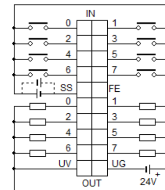
iR-DM16-N
