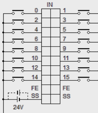
iR-DI16-K
