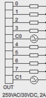
iR-DQ08-R
